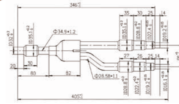
rura gazowa
