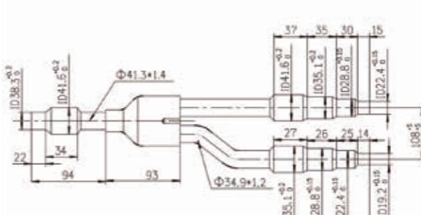
rura gazowa
