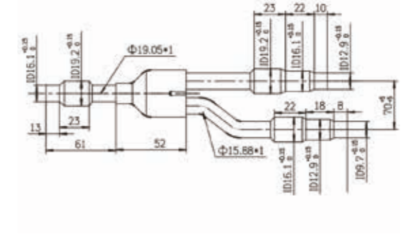
rura cieczowa
