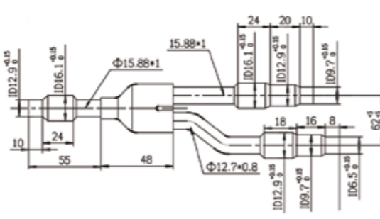
rura cieczowa
