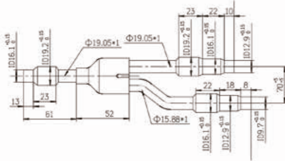
rura gazowa
